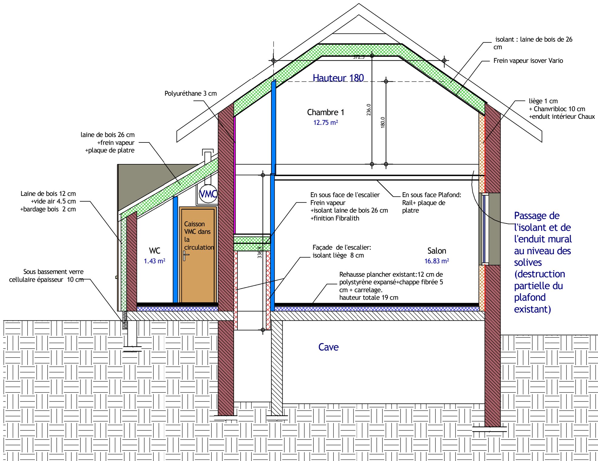
1 Coupe 1 Ech : 1 : 50
